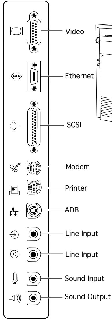
Macintosh Quadra 900/950
