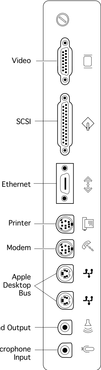
Macintosh Quadra 800
