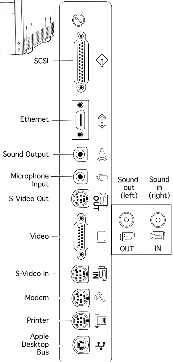
Macintosh Quadra 840AV
